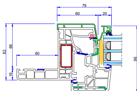
Telaio da ristrutturazione con aletta da 60 mm.
