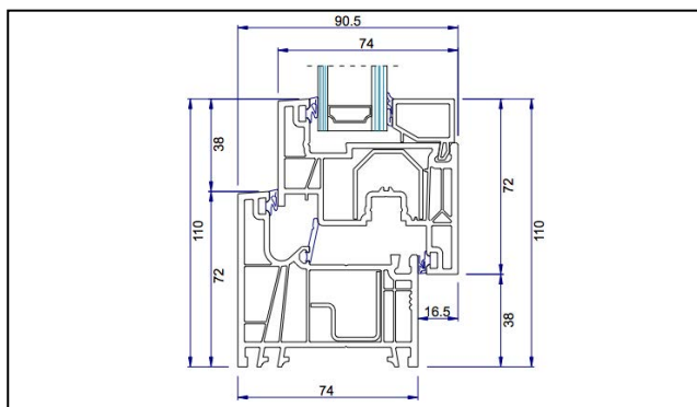
Nodo laterale simmetrico - 38 mm
