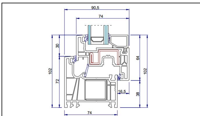
Nodo laterale asimmetrico - 30 mm
