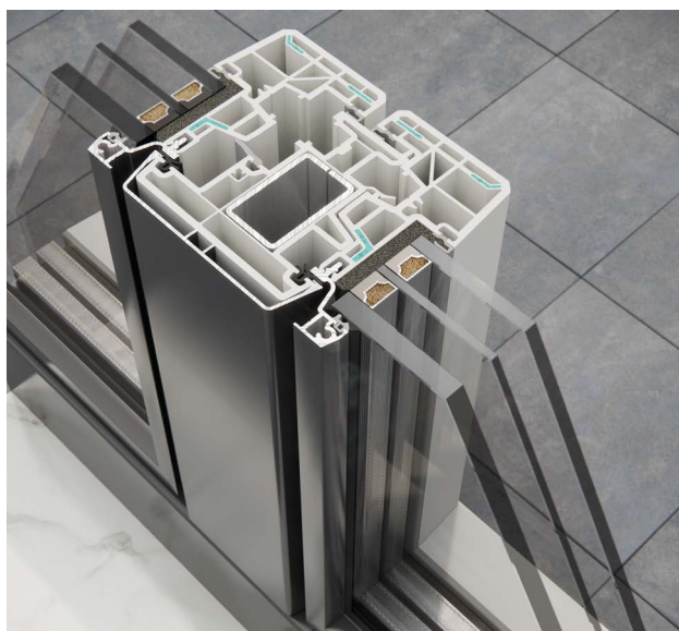
Nodo centrale simmetrico
