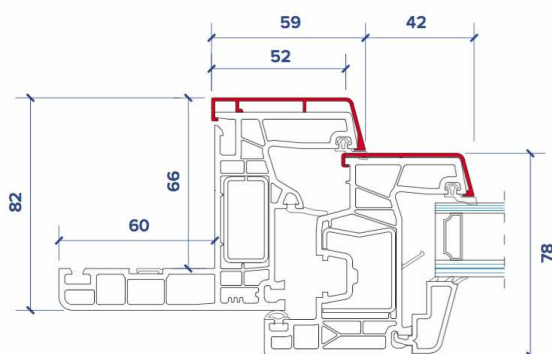
Telaio da ristrutturazione con aletta da 60 mm. Vista telaio parzialmente incassato dietro mazzetta.
