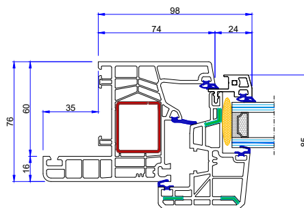
Telaio con aletta da 35 mm.
