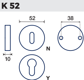
BOCCHETTA Ø 52 mm ESCUTCHEON Ø 52 mm
