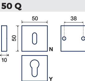
BOCCHETTA QUADRATA SQUARE ESCUTCHEON
